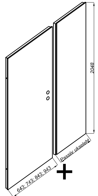
Puit profiillist
