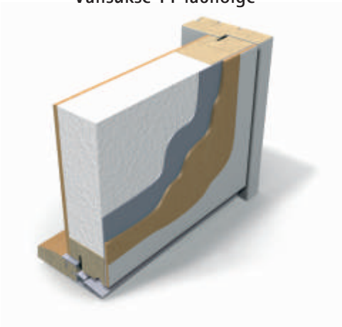
Välisukse T1 läbilõige
